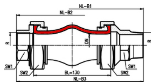
Megjegyzés | B1 típus (külső menetes) - gumikompenzátor | méretraajz
