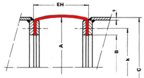
Megjegyzés | szövetkompenzátor - 45-ös típus | méretraajz
