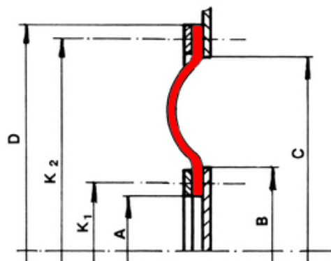
Megjegyzés | szövetkompenzátor - 35-ös típus | méretrajz
