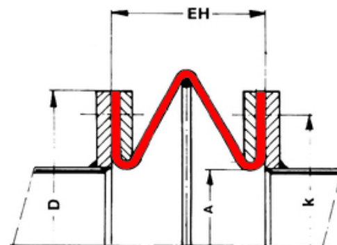
Megjegyzés | szövetkompenzátor - 33-as típus | méretrajz
