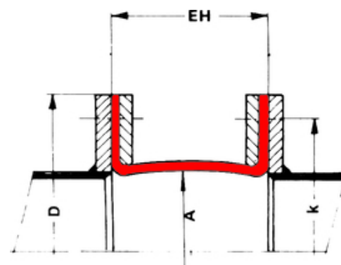
Megjegyzés | szövetkompenzátor - 31-es típus | méreterajz
