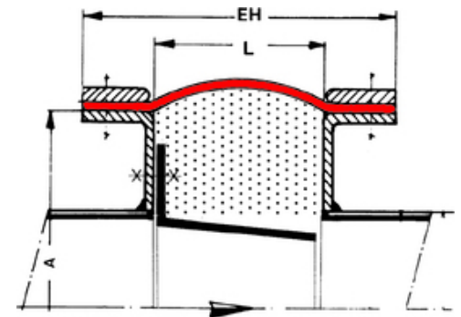
Megjegyzés | szövetkompenzátor - 22-es típus | méretrajz
